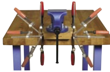
Schraubzwingen zum Anspannen nach unten drehen
